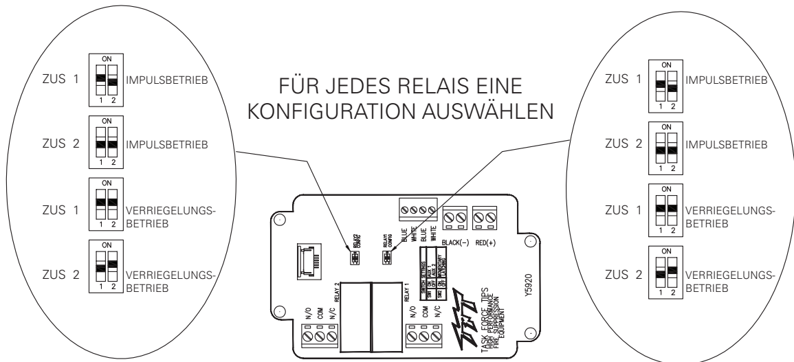
Abbildung 2.9.3 Relaiskonfiguration
