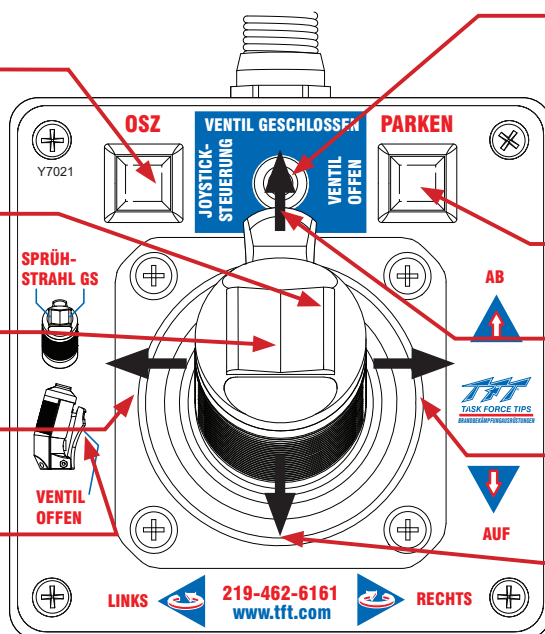
Abb. 2.5.3 Beschriftung am Joystick
