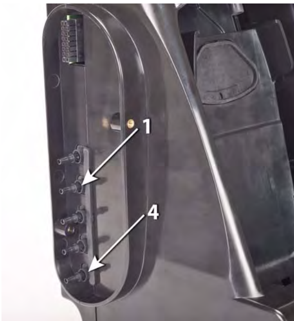
Bild 17 Gaseinlässe an der Prüfstation
